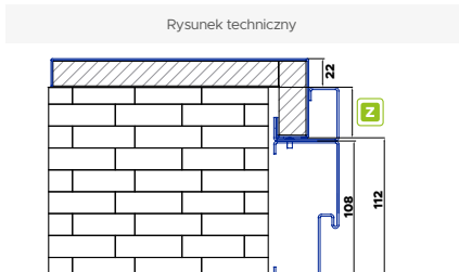
Złożenie ościeżnicy "11" Protect z łącznikiem portalu
