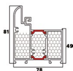
Rysunek techniczny
