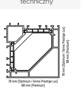
Rysunek techniczny
