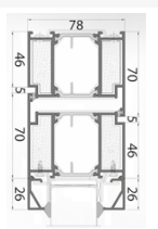
Rysunek techniczny
