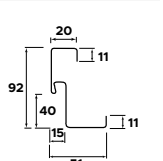
Rysunek techniczny
