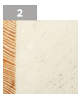
2 Skrzydło drzwiowe z uszczelką, wypełnione pianką poliuretanową oraz ramiakiem z drewna klejonego
