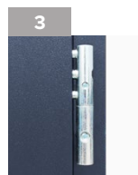
3 Trzy zawiasy 3D re- gulowane w trzech płaszczyznach
