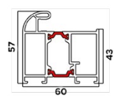
Rysunek techniczny
